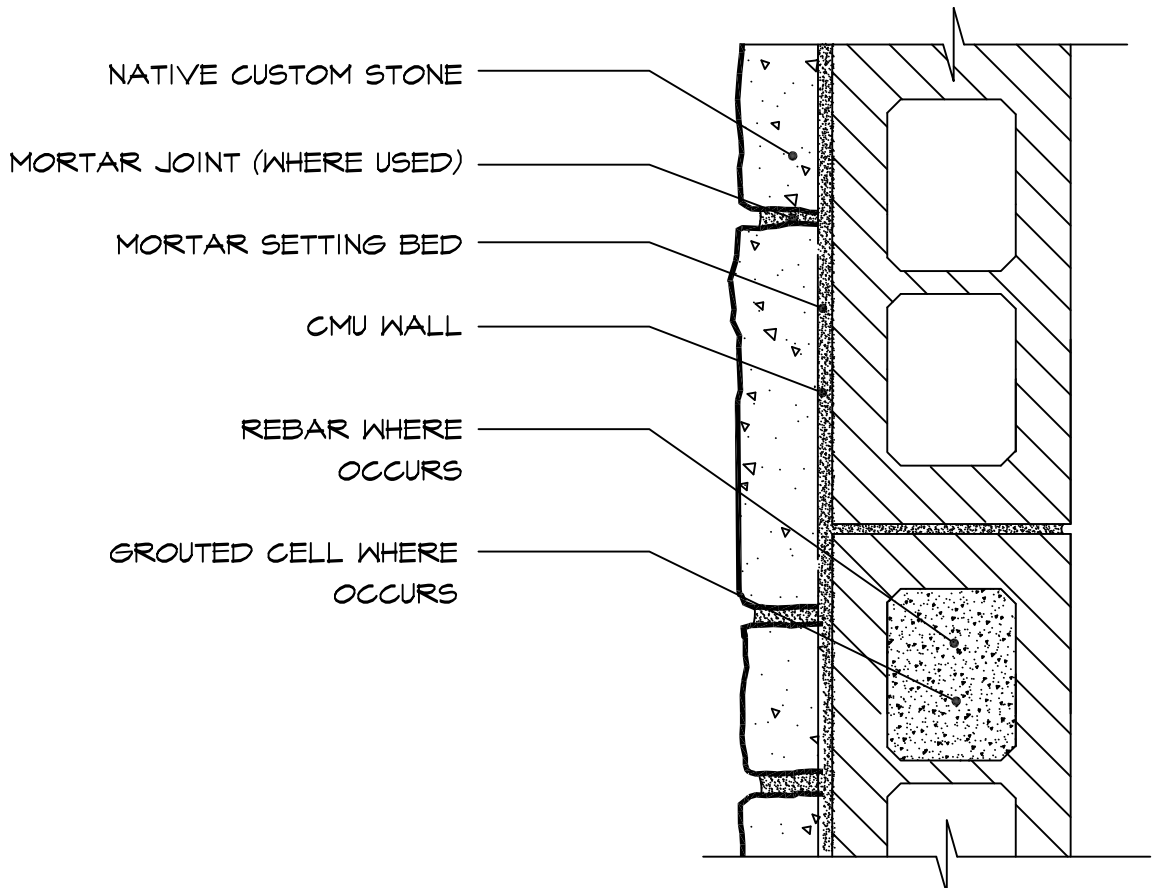
STONE @ CMU WALL SCALE: N.T.S.
