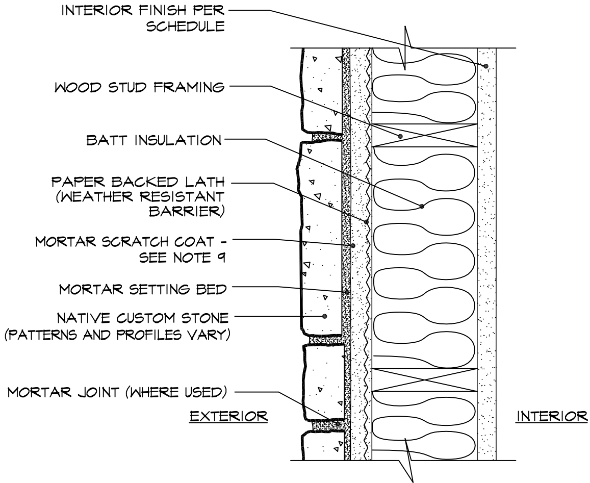
STONE OVER OPEN STUD FRAMING SCALE: N.T.S.
